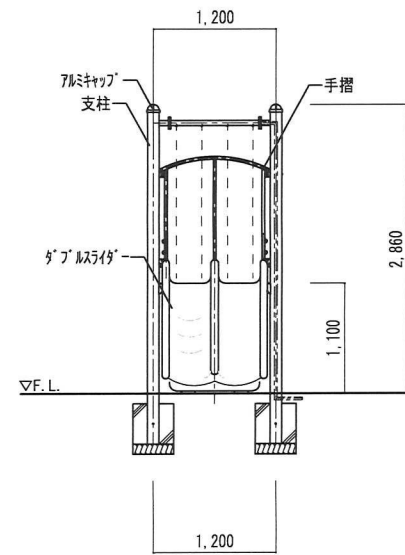
滑り台立面図 S:1/50
