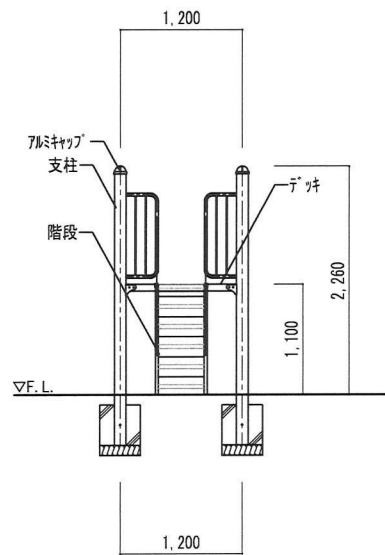
階段立面 S:1/50
