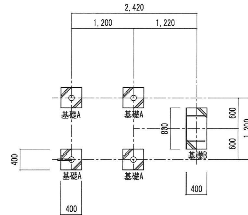
基礎伏図 S:1/50
