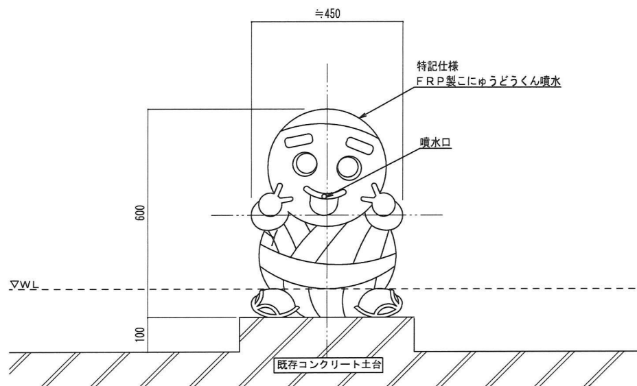
立面図 S:1/10
