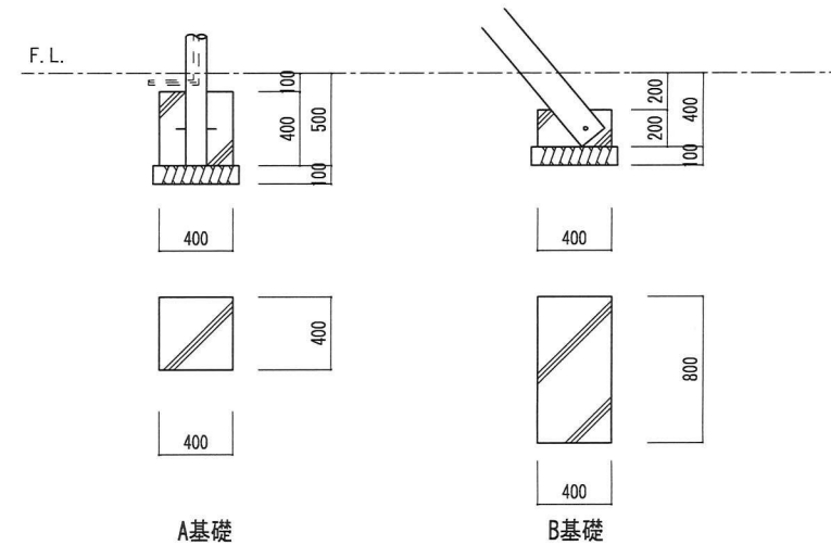
基礎詳細図 S:1/30
