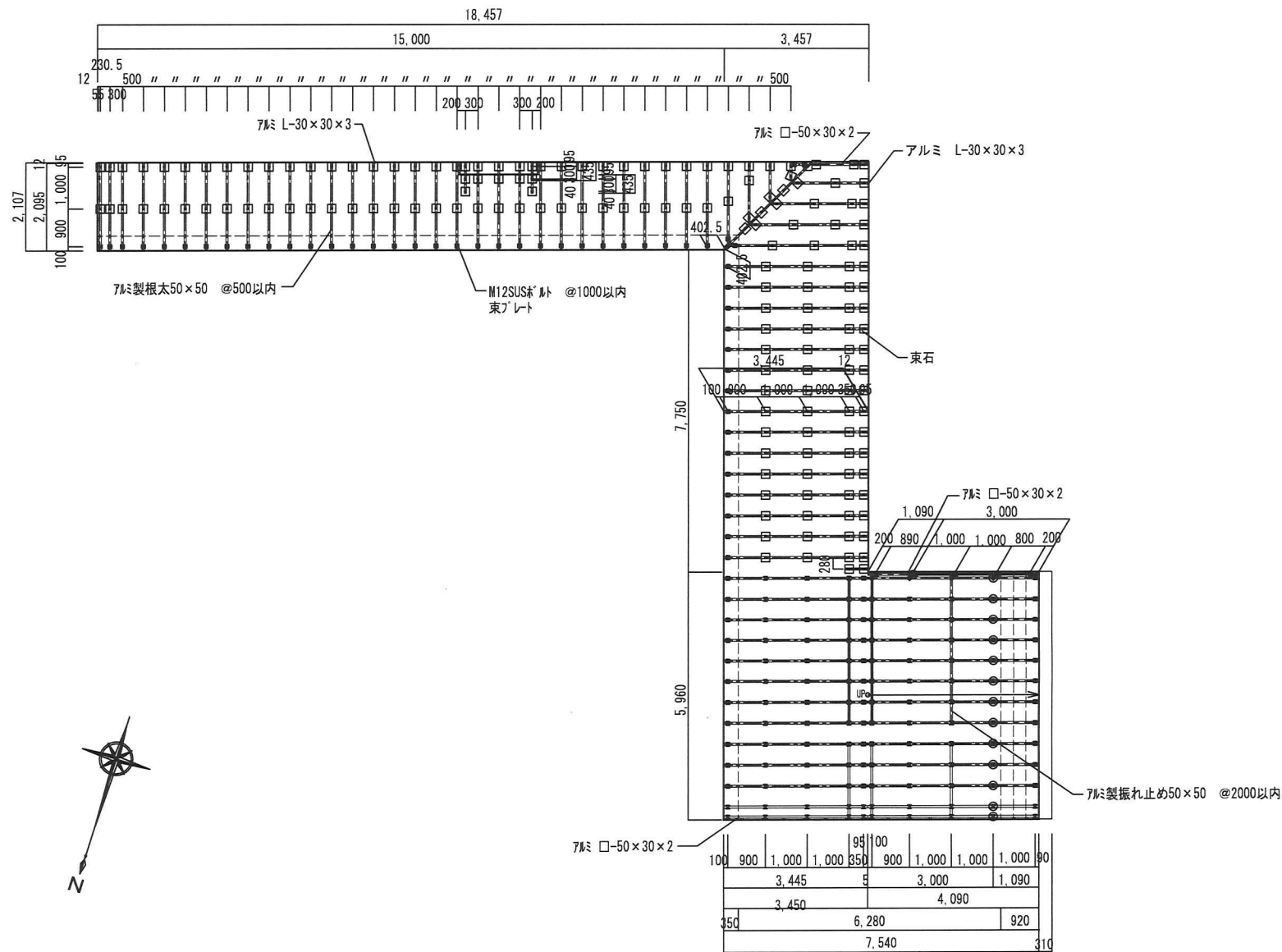
デッキ下地図 S:1/100
