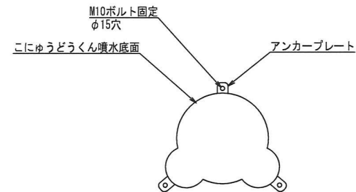
アンカープレート取付位置図 S:1/10
