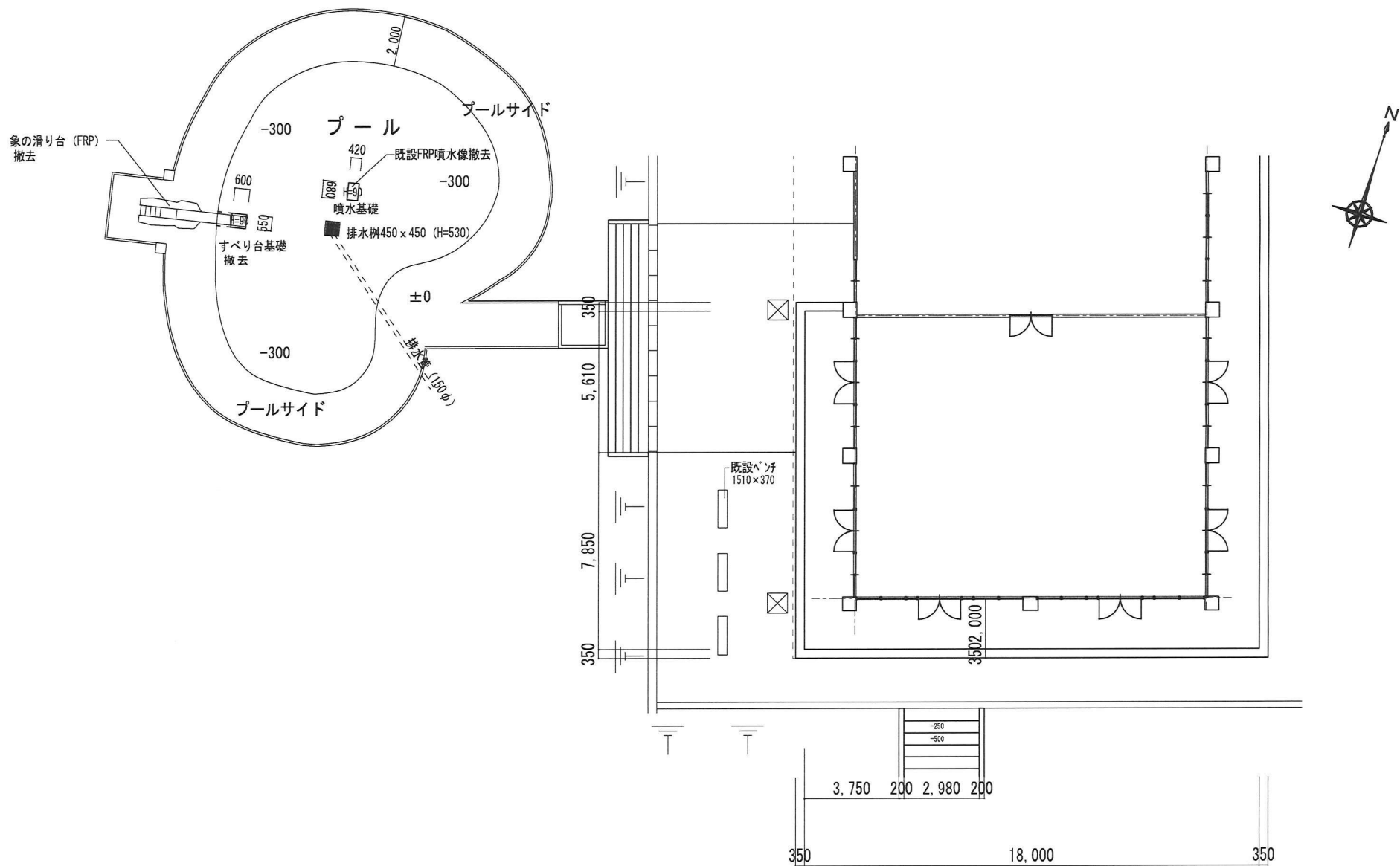
平面図 S:1/150
